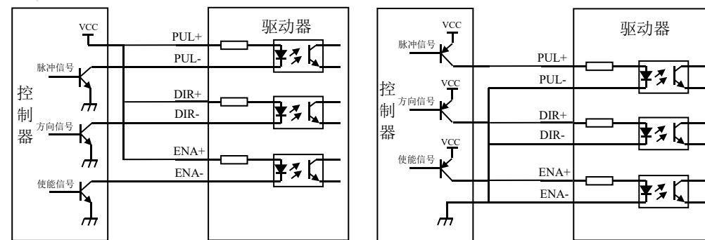
共阳极接法
